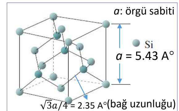
Silikon kristal birim hücresi (elmas yapı)
